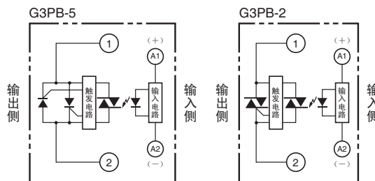
端子配置/内部接线
