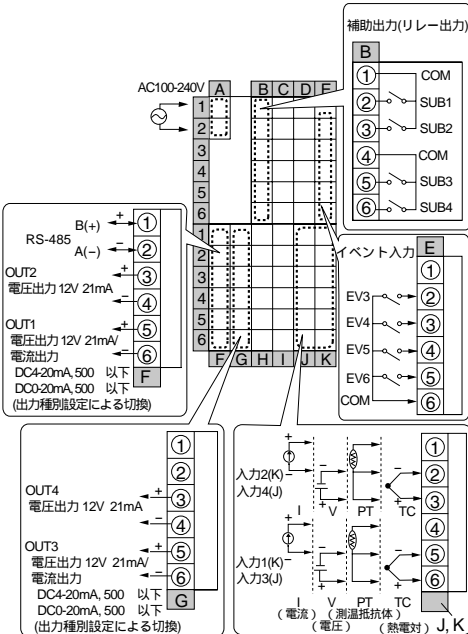
E5AR-QQ43DWW-FLK(4入力タイプ)
