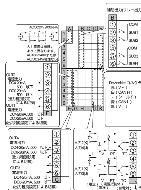
E5AR-CC4WW-DRT(4入カタイプ)
