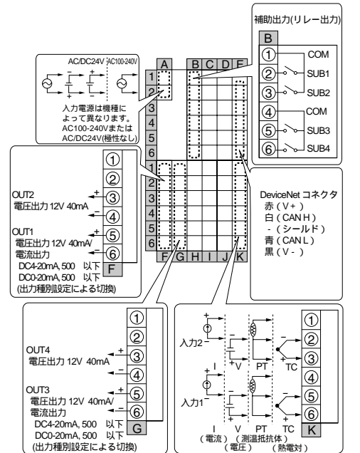
E5AR-QQ4W-DRT(2入カタイプ)
