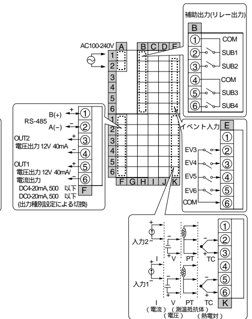
E5AR-Q43DW-FLK(2入力タイプ)
