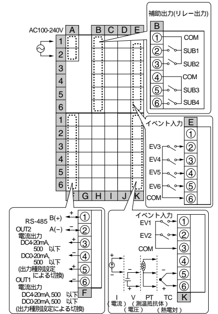
E5AR-Q43DW-FLK(2入力タイプ)
