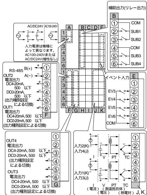
E5AR-CC43DWW-FLK(4入力タイプ)
