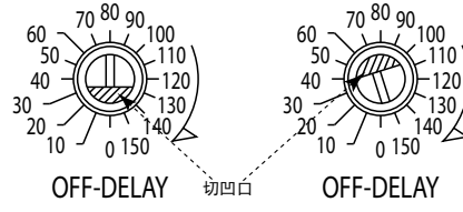
例1)关延迟时间0秒时 例2)关延迟时间70秒时
